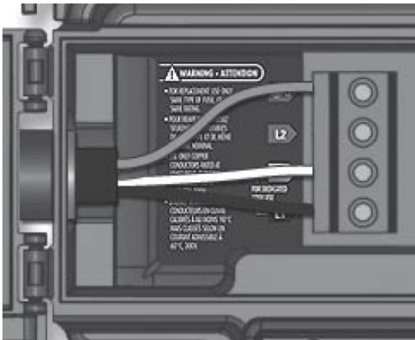
LEVITON - 120 VOLT TYPICAL
